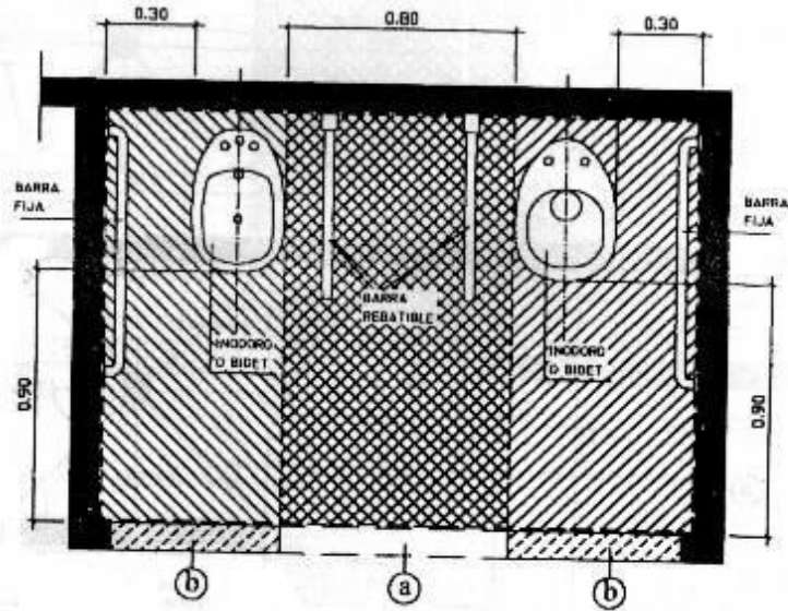
PLANTA
